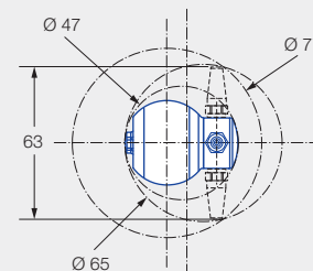
Einführdurchmesser und Störkreisdurchmesser
