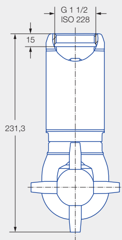
Innengewinde
