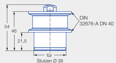
Tri-Clamp-Anschluss
