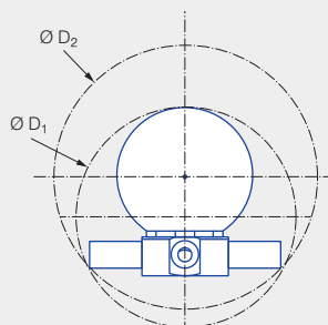
Einfuhrdurchmesser D_1 und Störkreisdurchmesser D_2 der Gewindeverbindung
