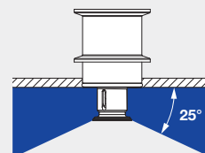
Tri-Clamp-Anschluss 2
