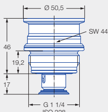
Außengewinde
