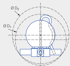
Einfuhrdurchmesser D_1 und Störkreisdurchmesser D_2 der Steckverbindung
