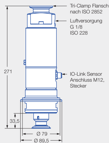
Tri-Clamp-Anschluss
