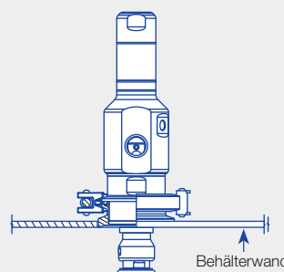
Tri-Clamp-Anschluss
