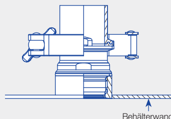
Gewindeanschluss
