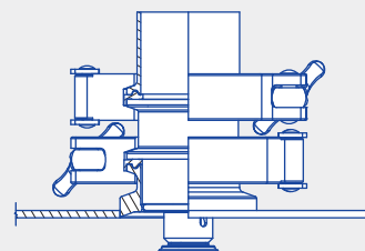
Tri-Clamp-Anschluss
