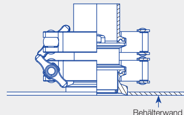
Tri-Clamp-Anschluss
