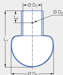
Abmessungen der Steckverbindung gemäß DIN 10357, Serie B
