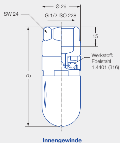
Innengewinde
