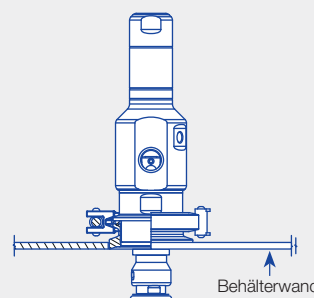
Tri-Clamp-Anschluss
