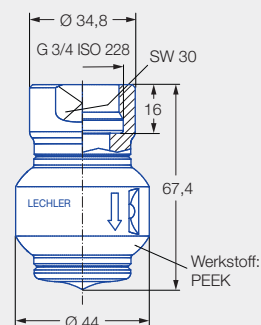
Innengewinde 595.139.1Y.AL
