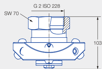
Innengewinde
