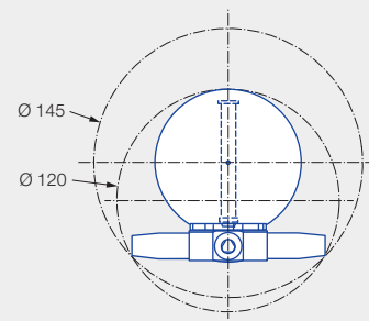
Einführdurchmesser und Störkreisdurchmesser der Steckverbindung
