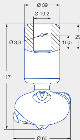
Abmessungen der Steckverbindung gemäß ASME-BPE (OD-Tube)
