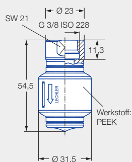
Innengewinde 59x.xx9.1Y.AF
